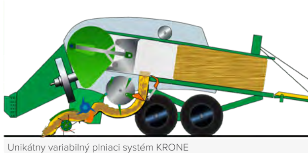
Unikátny variabilný plniaci systém KRONE
