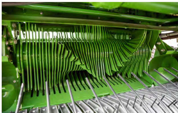
Maximálne výkonné lisy KRONE aj kvôli rezaciemu rotoru aj s meniteľným počtom nožov
