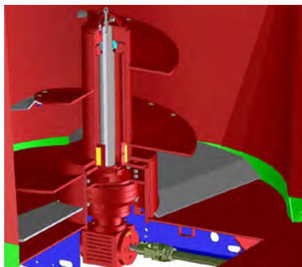
Vertikálny systém miešania s jednou závitovkou na kŕmnom voze SOLOMIX 1
