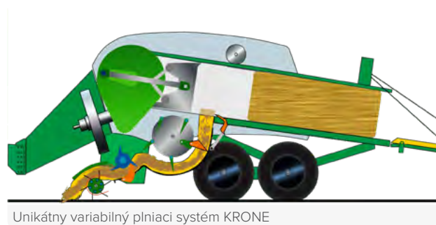
Unikátny variabilný plniaci systém KRONE
