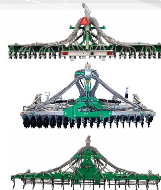
Možnosti rôznych aplikátorov na cisterny SAMSON - bezstratová a rovnomerná aplikácia
