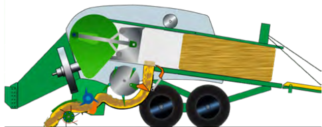
Unikátny variabilný plniaci systém KRONE
