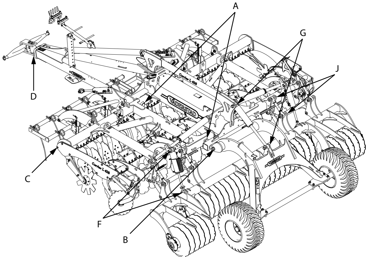
Obrázek 9.4 Na obrázku je stroj CRL 425 s bránami na slámu a nosníkem tažné oje.
