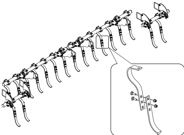
Obrázek 7.20 Výškové nastavení prstu urovnávací jednotky
