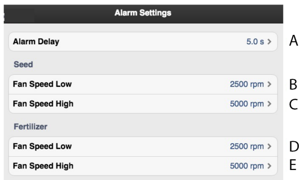
Obrázek 6.18 Nastavení alarmů v menu iPadu
