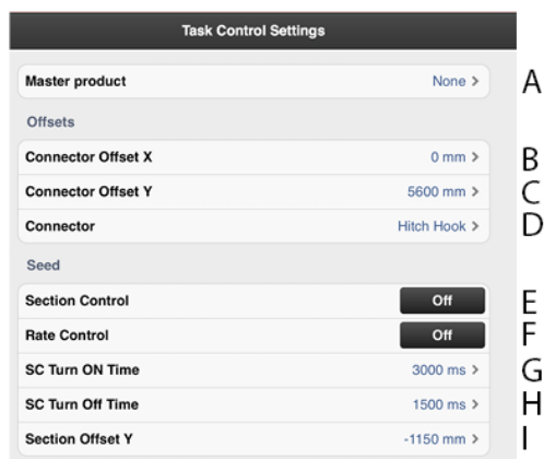
Obrázek 6.7 Nastavení ISOBUS Task Control
