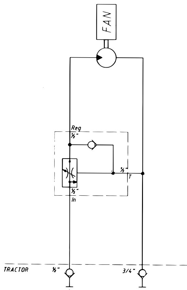
Obrázek 12.2 Hydraulické schéma ventilátoru, sériové číslo -180
